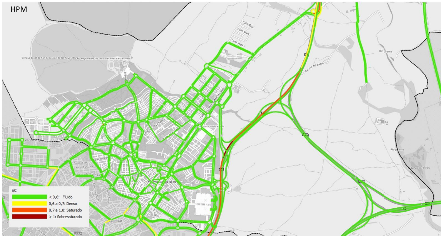
Ilustración 64. Mapa de I/C en hora punta de mañana (nivel de saturación). Fuente: Elaboración propia
