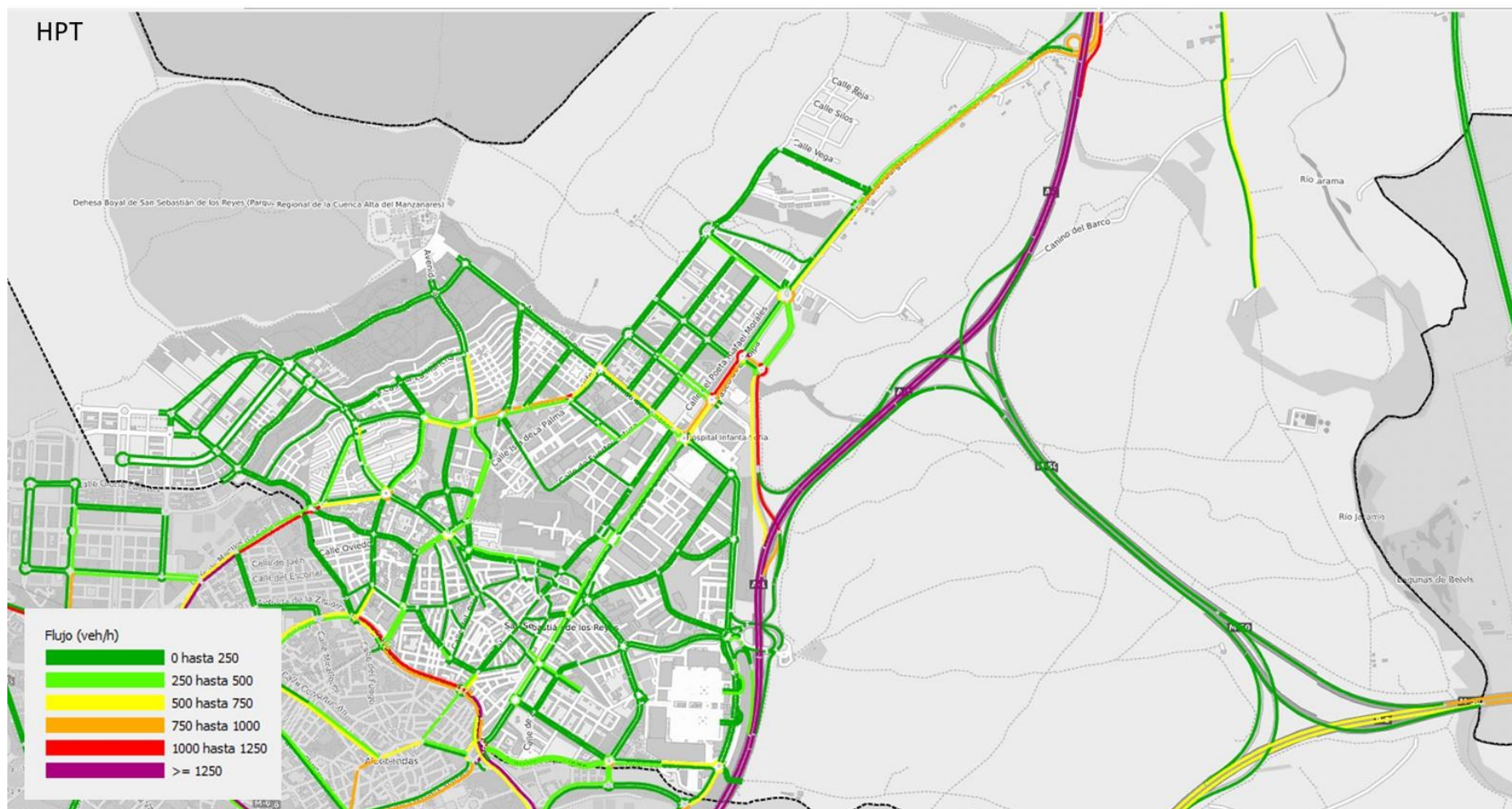
Ilustración 63. Intensidades en hora punta de tarde. Fuente: Elaboración propia
